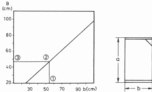
Diagramm 11: Form B3, Ventillachsack befüllt – Maße A und B
