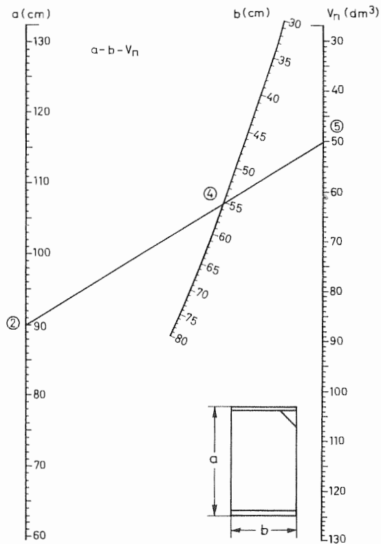
Nomogramm 12: Form B3, Ventilflachsack - 30 bis 130 dm 3
