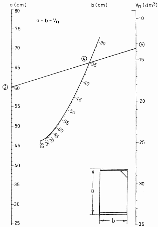
Nomogramm 11: Form B3, Ventilflachsack - 10 bis 35 dm 3
