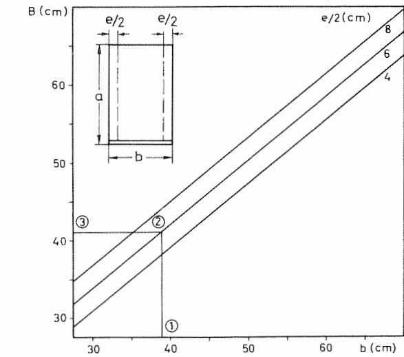
Diagramm 3: Form A2, Faltensack befüllt – Maße A und B
