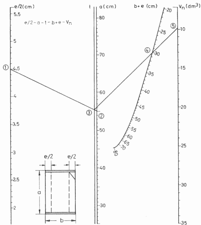
Nomogramm 9: Form B2, Ventilfaltensack – 10 bis 35 dm 3
