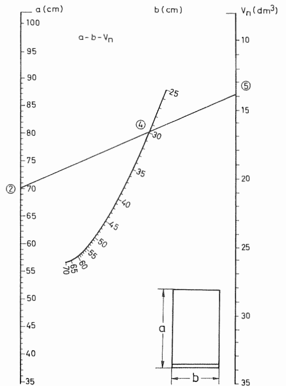
Nomogramm 5: Form A4, Flachsack – 10 bis 35 dm 3
